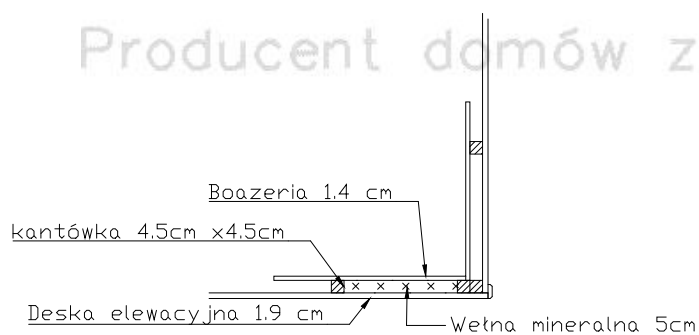
Szczegół przekrój ściana zewnętrzna
