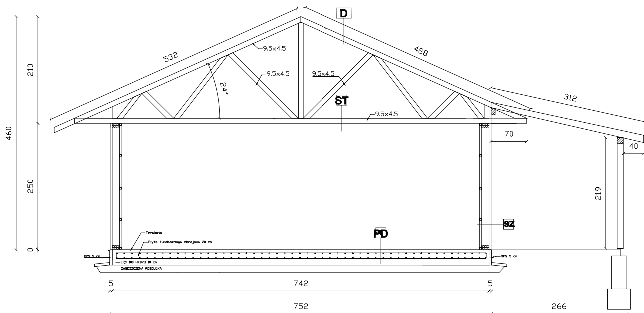
Przekrój
