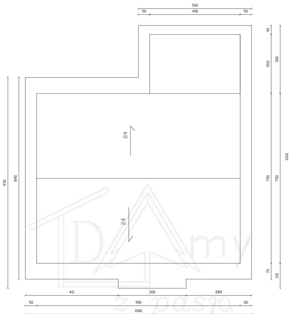
Rzut dachu
